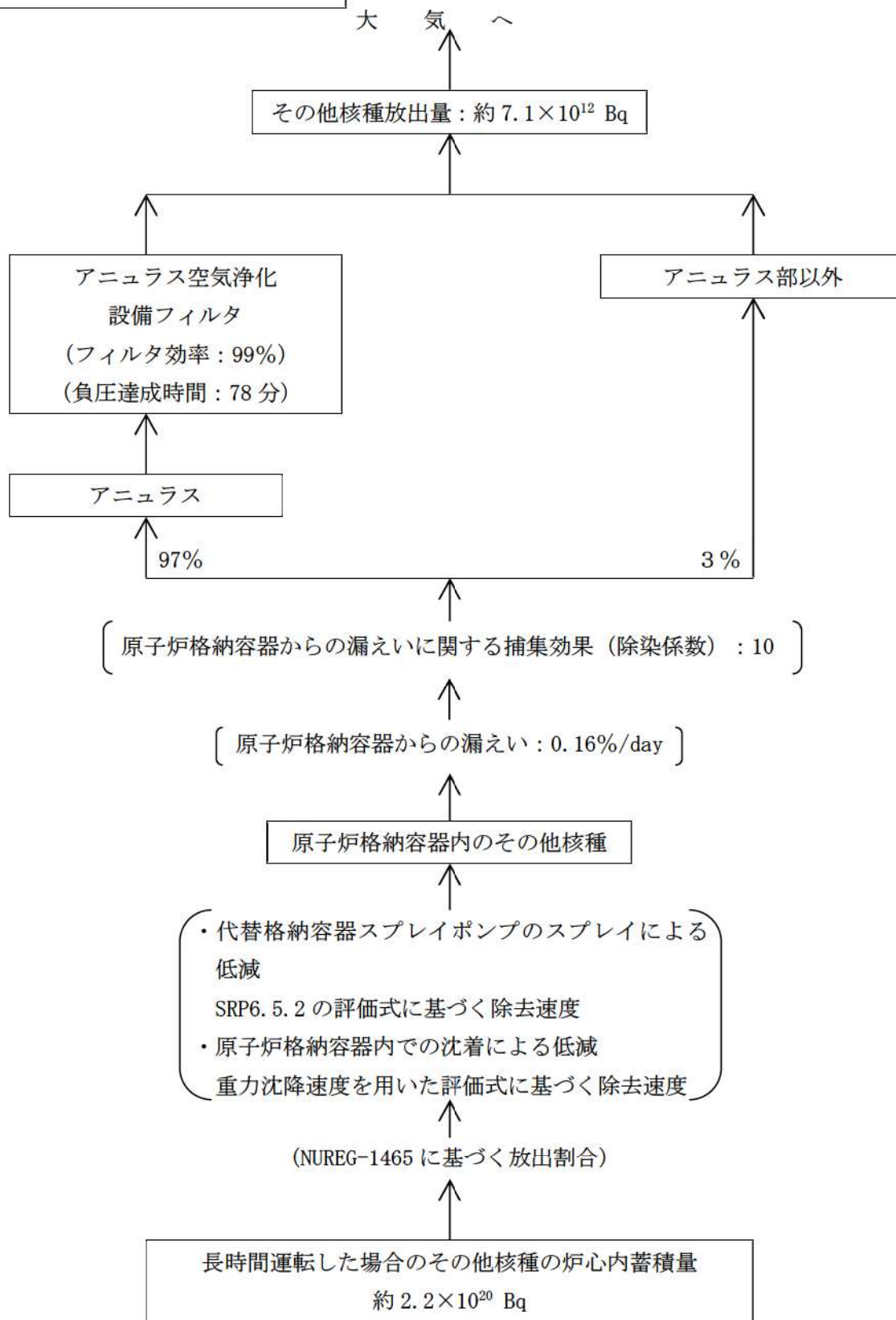
第 2-5-7 図 その他核種の大気放出過程
