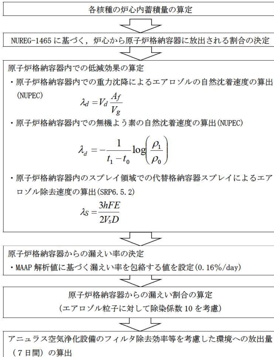
第 2-5-2 図 大気中への放出放射能量算定の概略フロー
