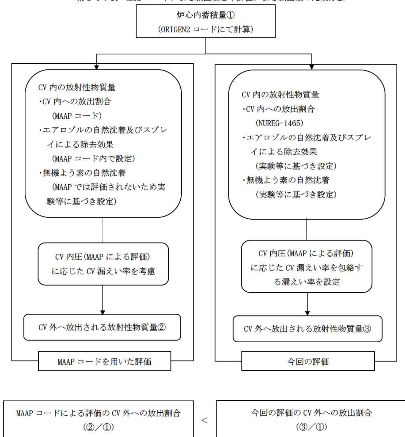
第 2-4-9 表 MAAP コードによる放出量と本評価による放出量の比較方法
