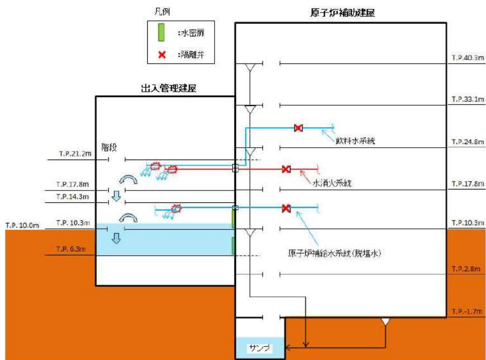
図 11-1 出入管理建屋の溢水概念図
