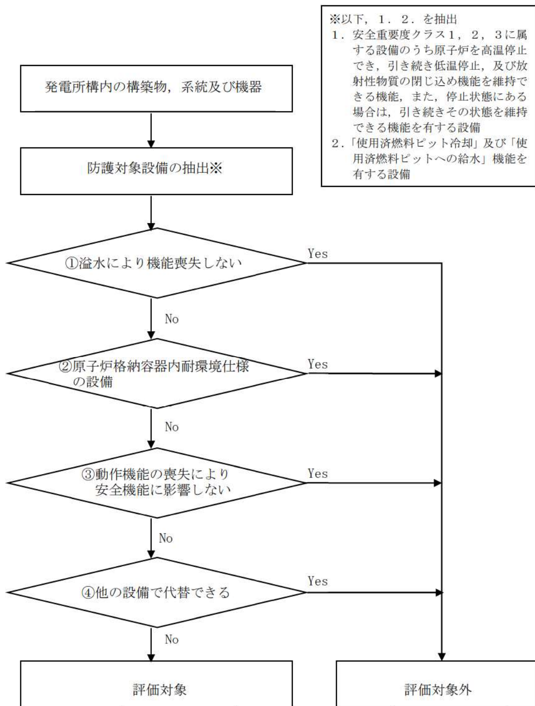
図 3-1 防護対象設備のうち洪水影響評価対象の選定フロー
