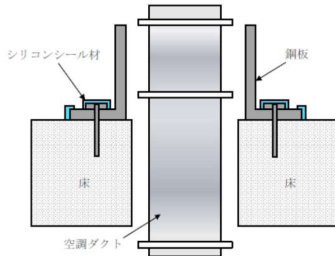
図2 ダクトに対する溢水対策
