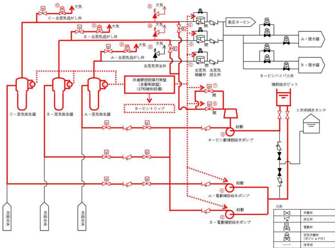
図 44-4-3 原子炉出力抑制（2）
