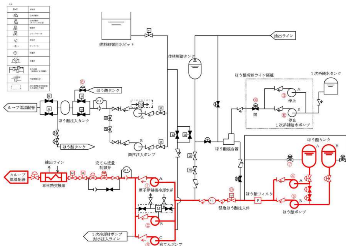
図 44-4-5 ほう酸水注入 (1)
