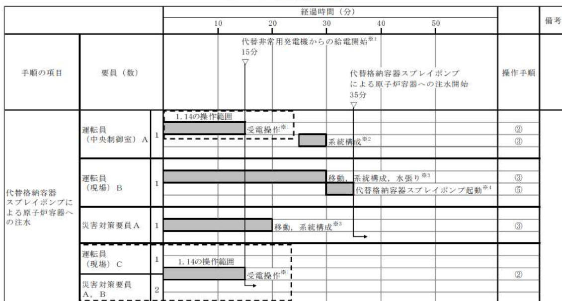
図 2.4-2 代替炉心注水 (代替格納容器スプレイポンプ) のタイムチャート (フロント系故障時) ※
