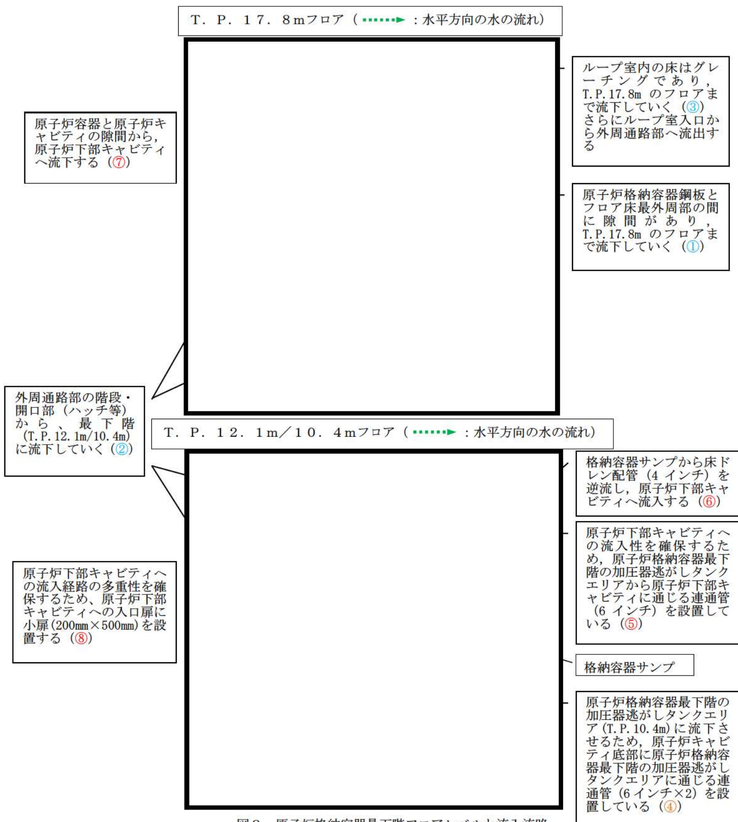
図8 原子炉格納容器最下階フロアレベルと流入流路
