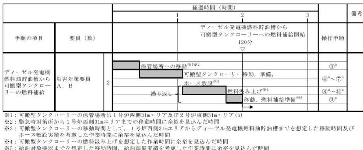
図 2.14.7 ディーゼル発電機燃料油貯油槽から 可搬型タンクローリーへの燃料補給のタイムチャート（ホース使用時）*
