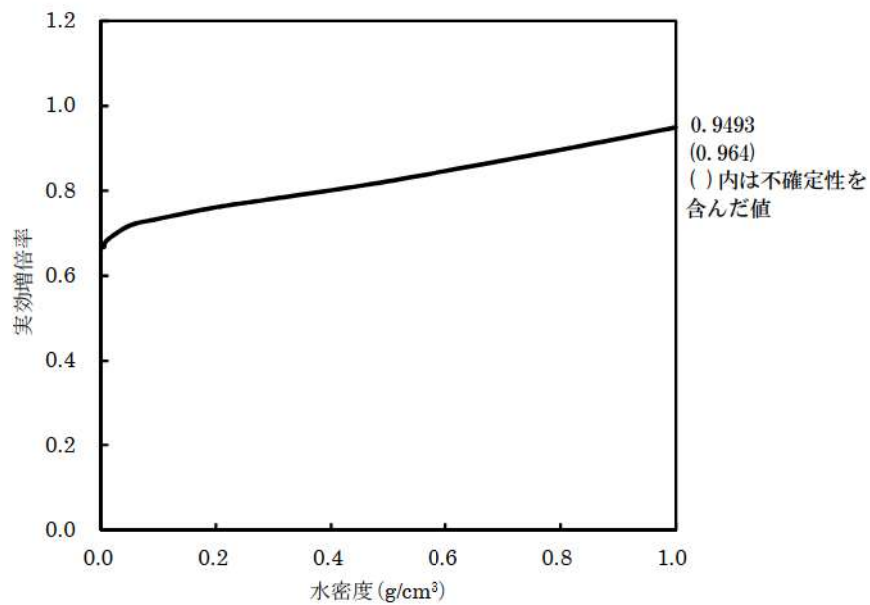
第6図 Bー使用済燃料ピットにウラン新燃料のみを貯蔵した場合の実効増倍率と水密度の関係（有限配列体系）
