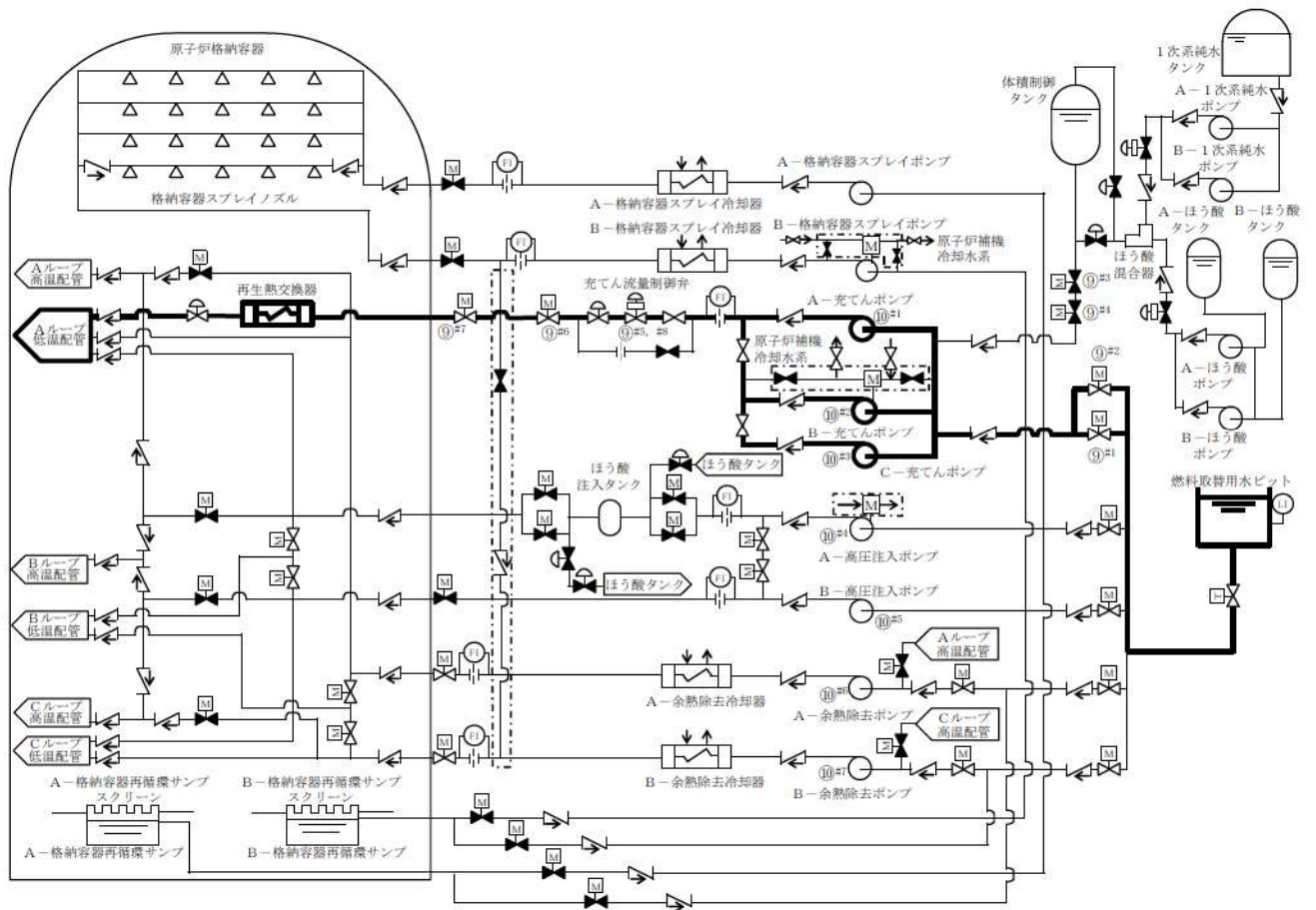
第 1.4.20 図 格納容器再循環サンプスクリーン閉塞の兆候が見られた場合の手順 (燃料取替用水ピットを水源とした充電ポンプによる原子炉容器 への注水) 概要図 (1/2)
