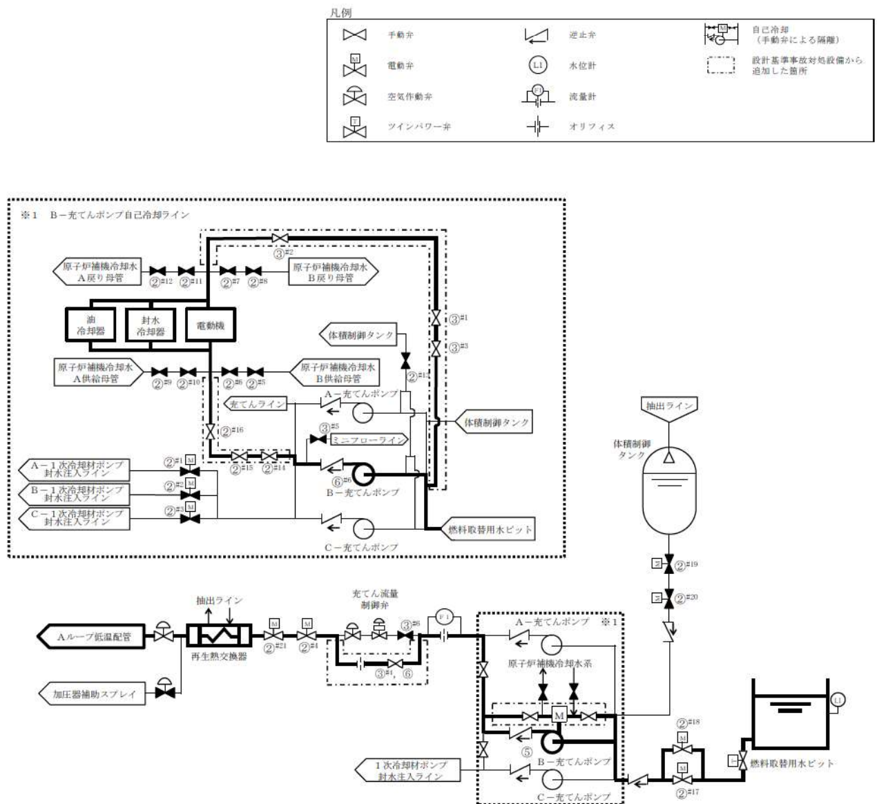
第 1.4.22 図 B-充てんポンプ（自己冷却）による原子炉容器への注水 概要図（1/2）
