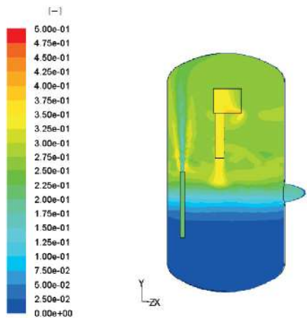
図 2.48 ST4-1 試験 DW1-ヘリウムモル分布 (2,000 秒、Phase2)
