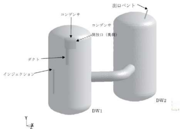
ST4-1 試験解析モデル（ダクト有り上段配置）
