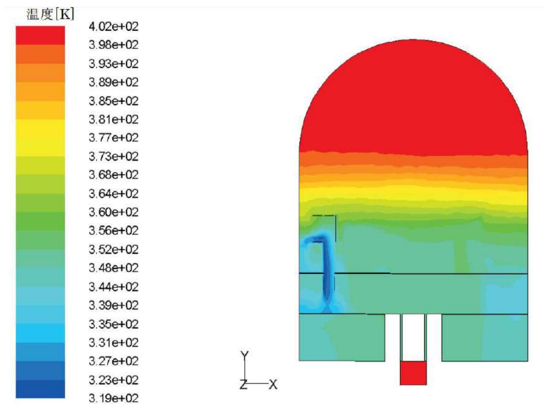
図 10 温度分布 (3600 秒, ループ室破断)
