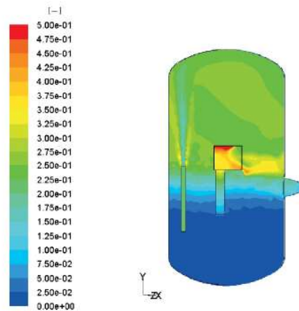
図 2.49 ST4-2 試験 DW1-ヘリウムモル分布 (2,000 秒、Phase2)
