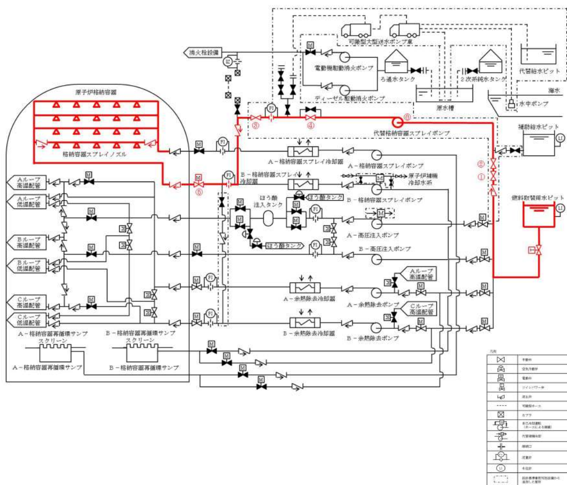
図 49-4-2 代替格納容器スプレイ
