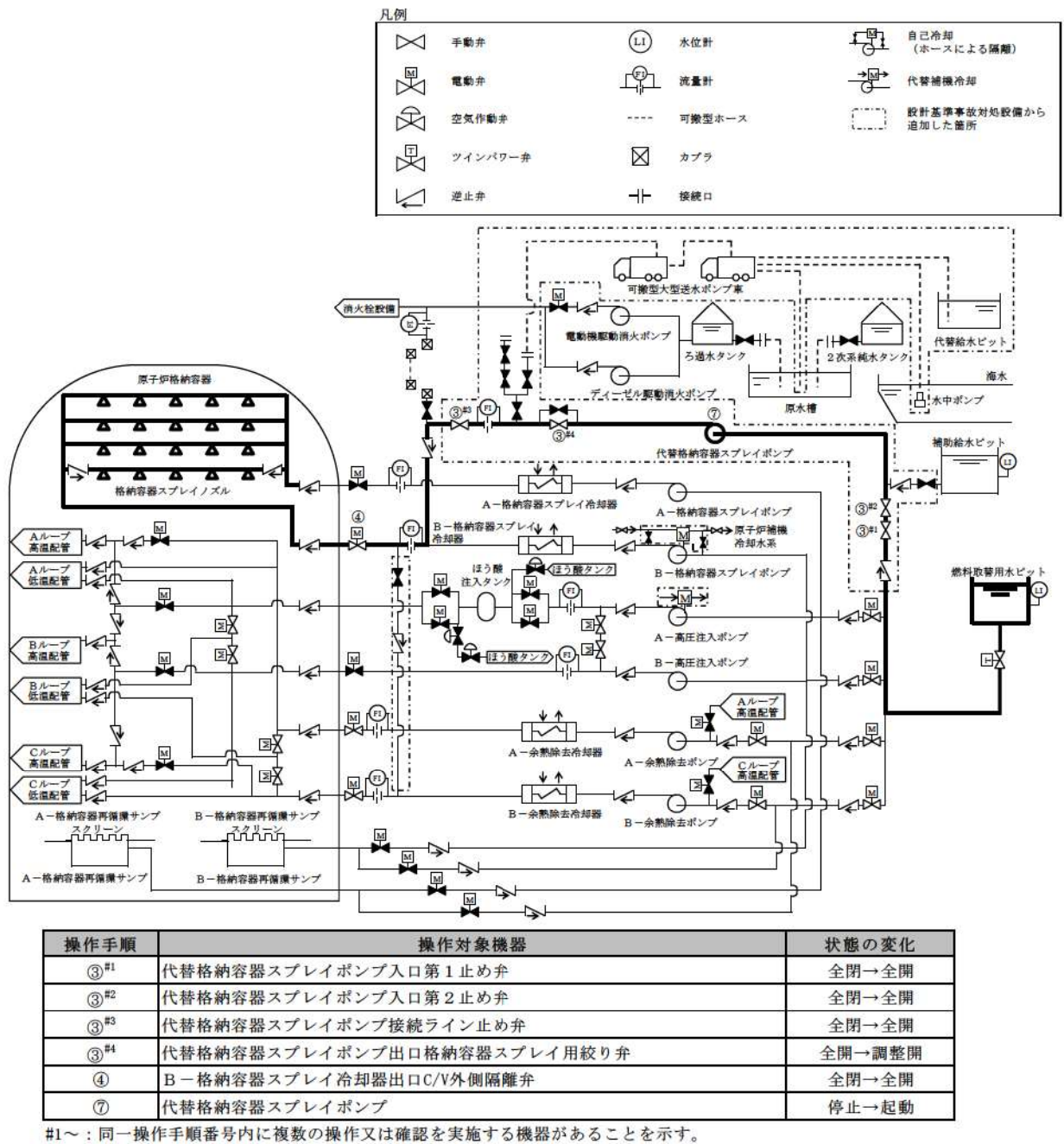
第 1.8.3 図 代替格納容器スプレイポンプによる原子炉格納容器下部への注水 概要図
