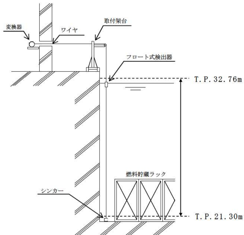
第４図 使用済燃料ピット水位（可搬型）の計測範囲
