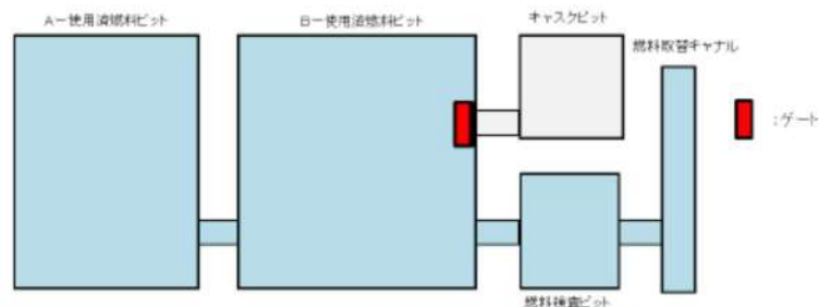
図1 使用済燃料ピット概略図 (平面図)
