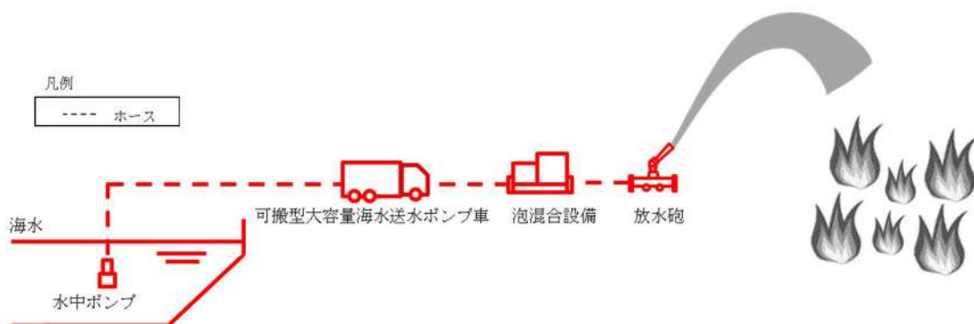
図 2.12-7 放水設備（泡消火設備）
