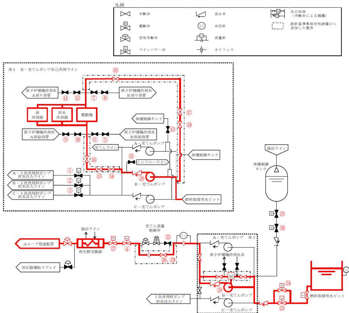
図4 B-充てんポンプ（自己冷却）による原子炉容器への注水 概要図
