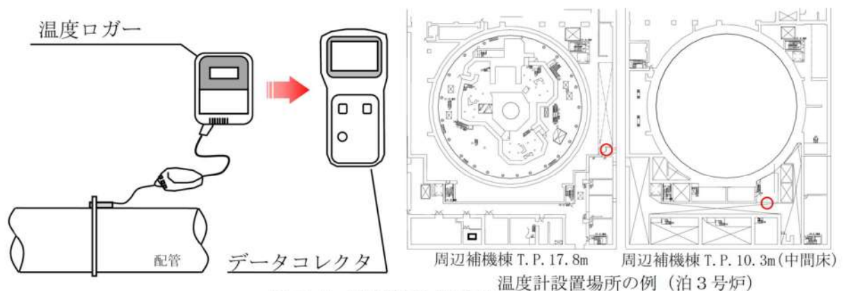
第1図 温度計取付け模式図
