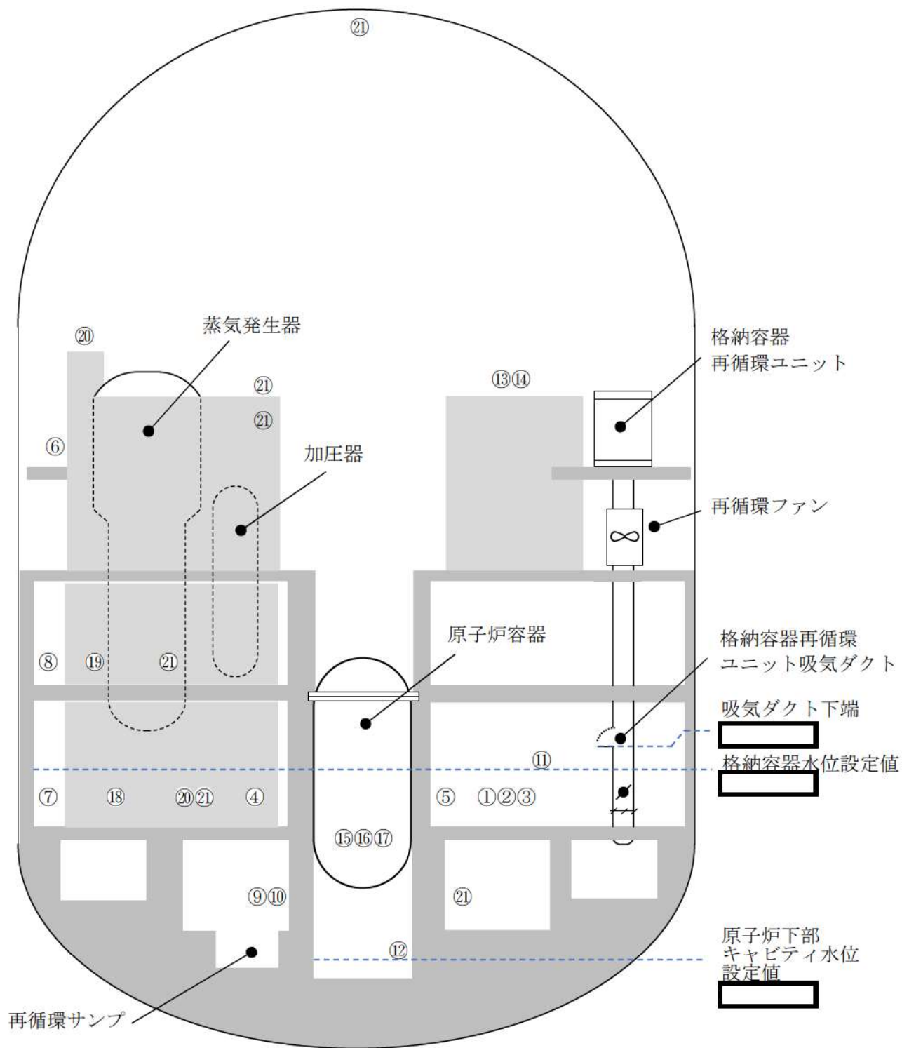
第 1 図 概略系統図
