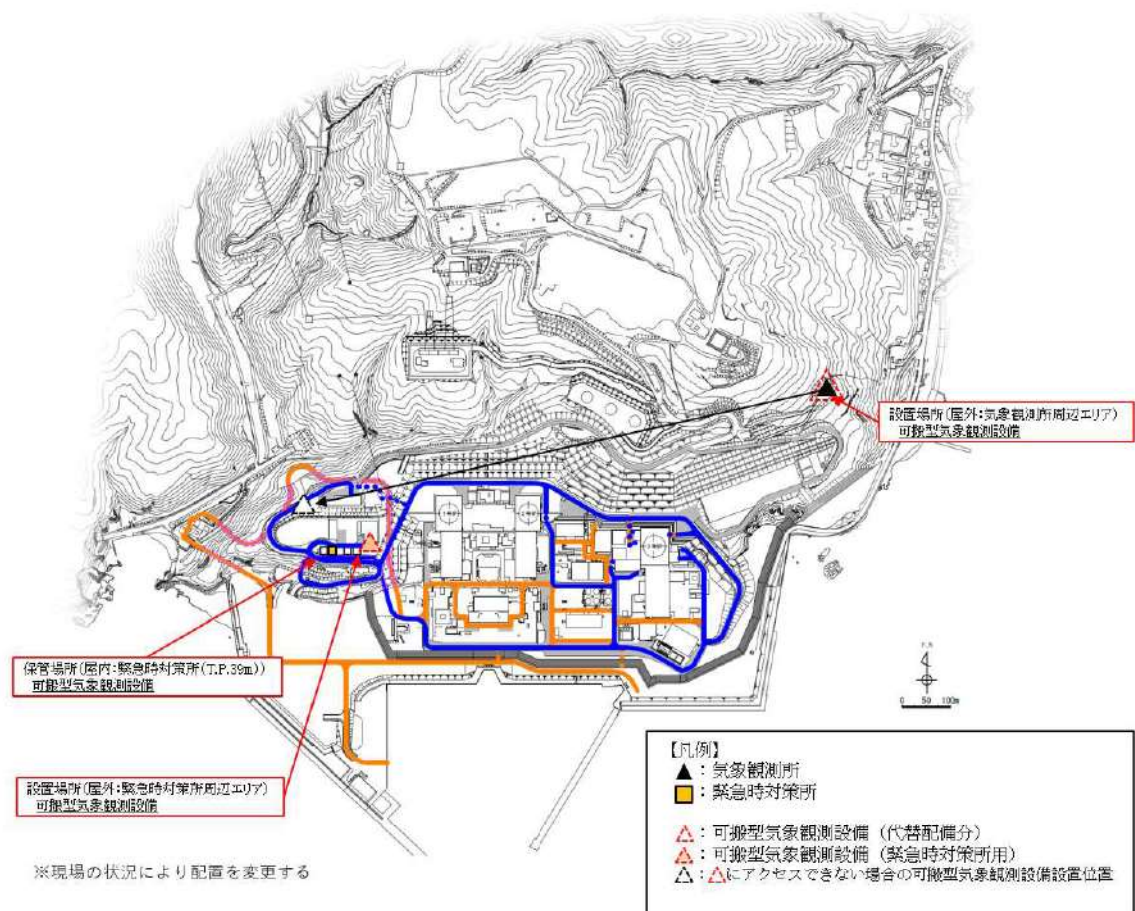
図1 可搬型気象観測設備の設置場所及び保管場所
