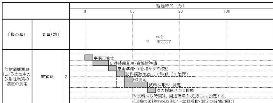
第1.17.6図 放射能観測車による空気中の放射性物質の濃度の測定 タイムチャート
