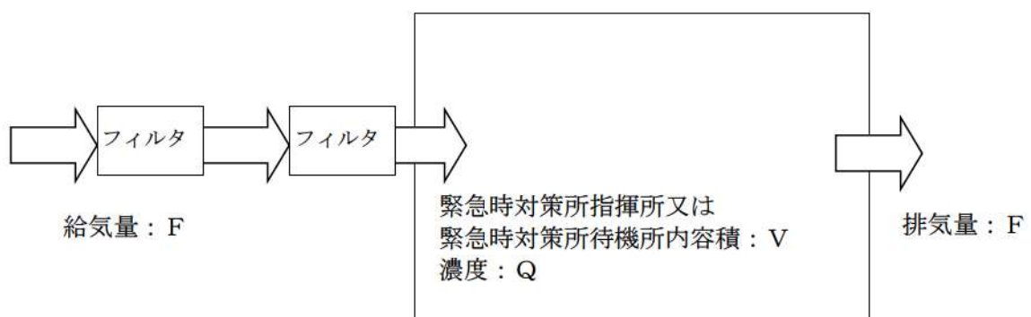
図添 10-2 濃度評価モデル(完全混合ボックスモデル)
