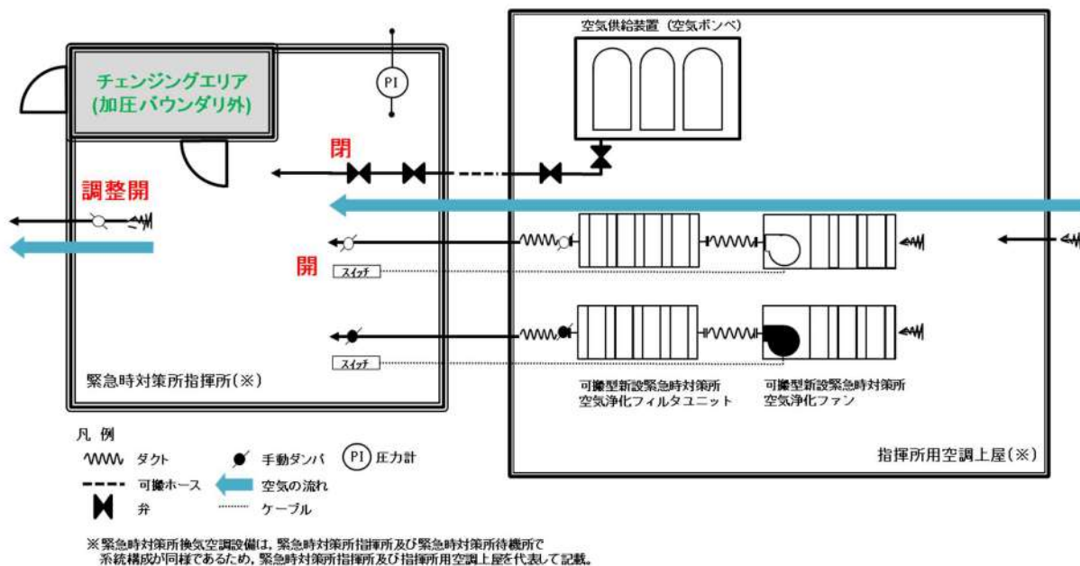
図2.4-1 緊急時対策所換気空調設備 系統概要図 (プルーム通過前及び通過後：可搬型新設緊急時対策所空気浄化ファンによる正圧化)
