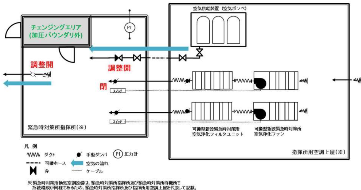
図2.4-2 緊急時対策所換気空調設備 系統概要図 (プルーム通過中：空気供給装置 (空気ポンプ) による正圧化)
