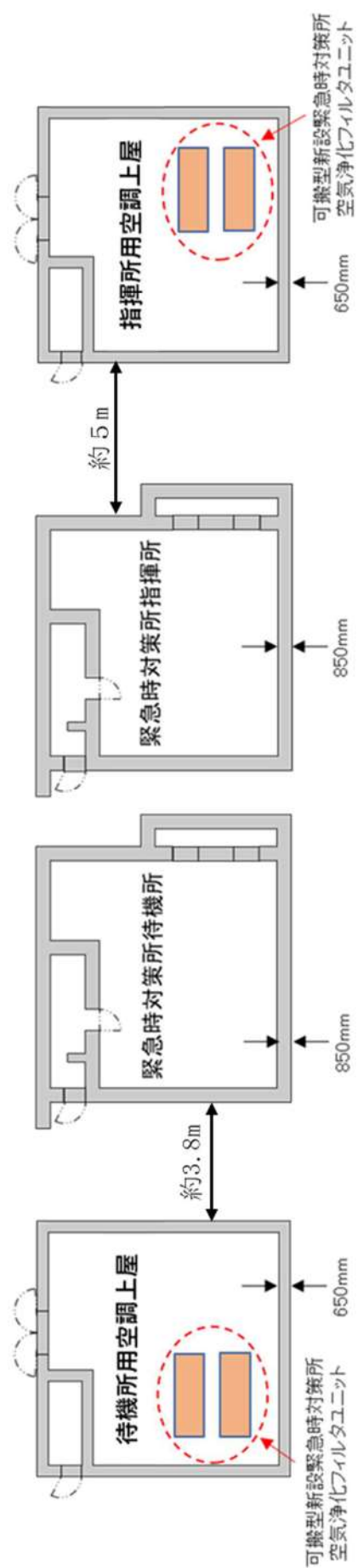
図2.4-23 可搬型緊急時対策所空気浄化ファン及びフィルタユニット設置位置
