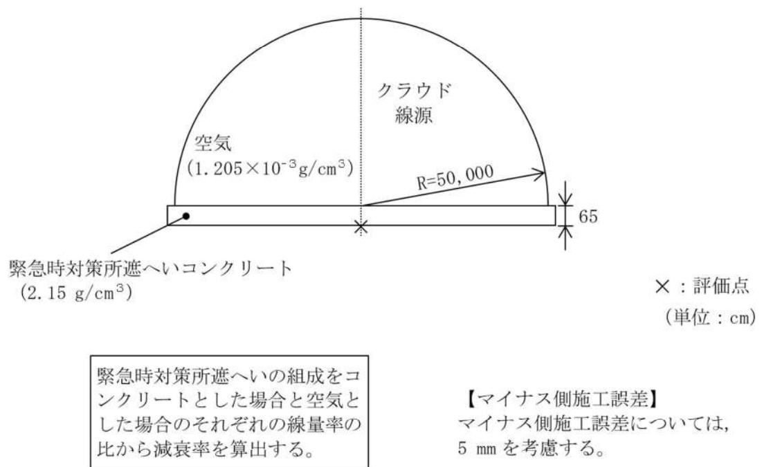
図添 8-1 クラウドシャインガンマ線に対する緊急時対策所遮へいによる減衰率計算モデル
