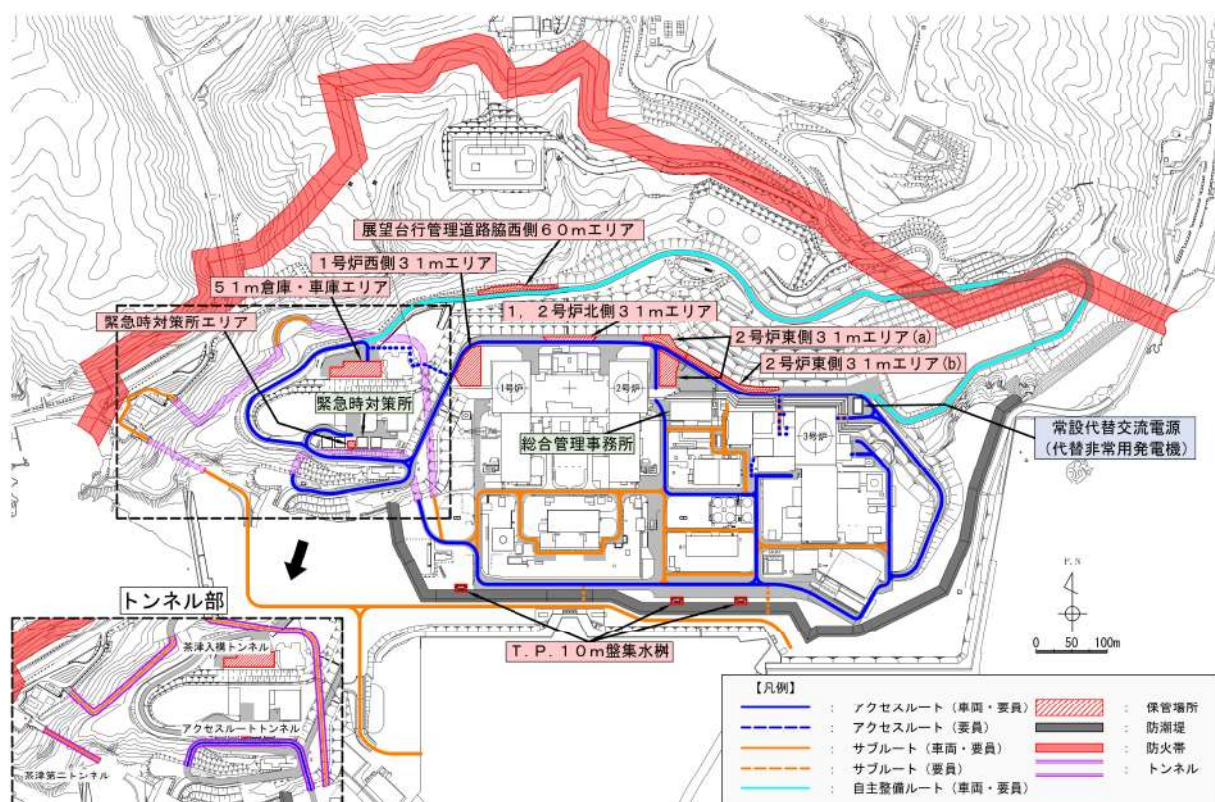
第2図 保管場所及び屋外アクセスルート図 (令和4年12月6日説明時点)
