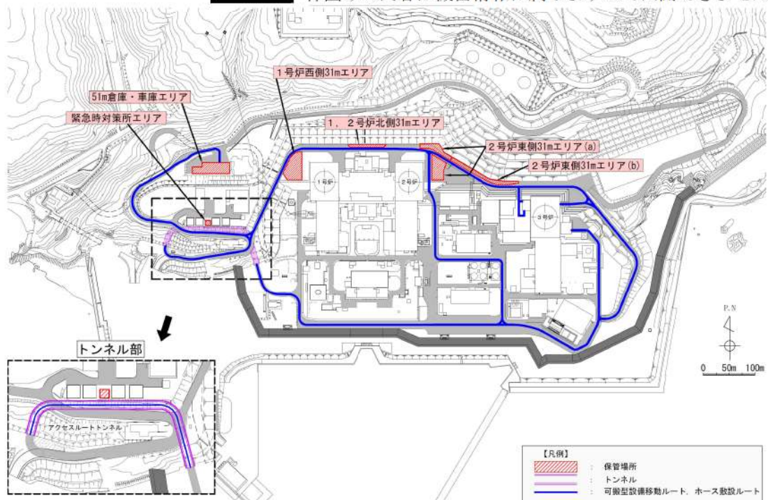
第5図 可搬型大型送水ポンプ車による注水
