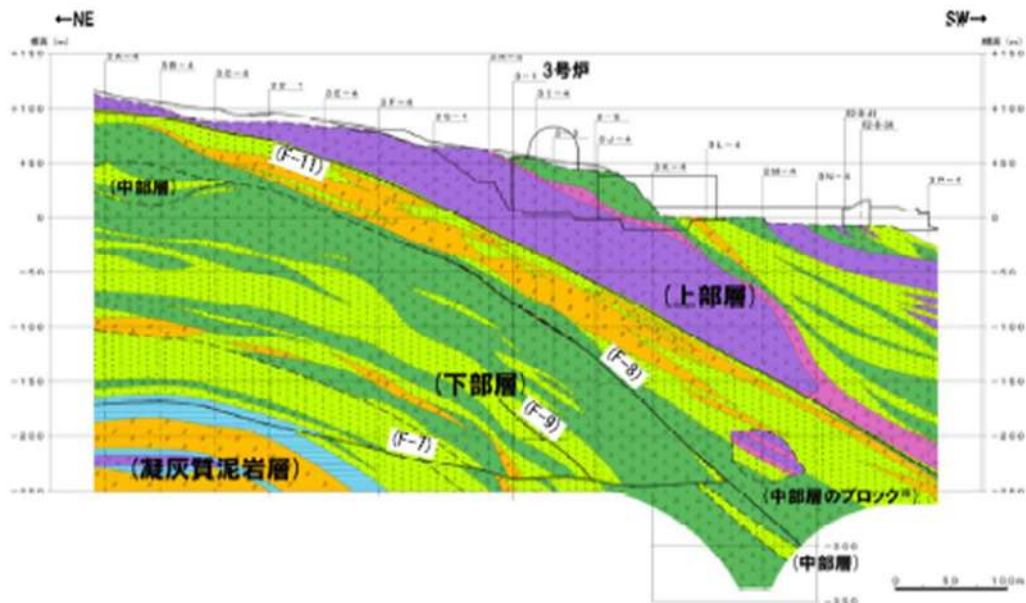
Y3-Y3' 断面
