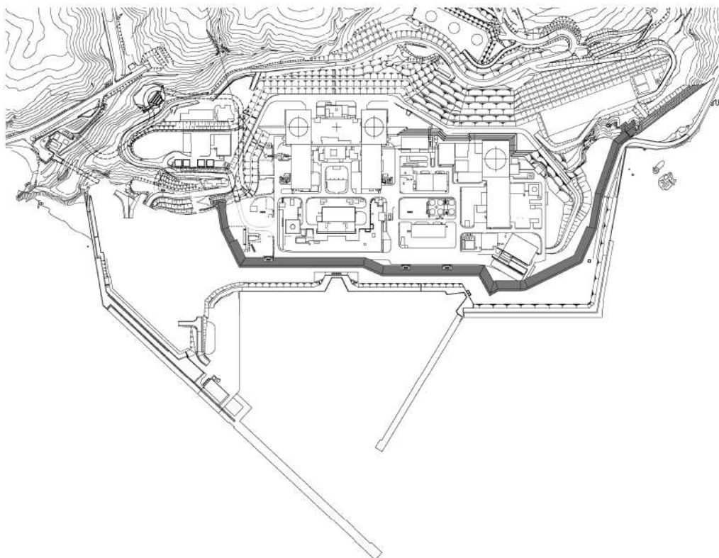
図 1.1.a.c-4 敷地平面図
