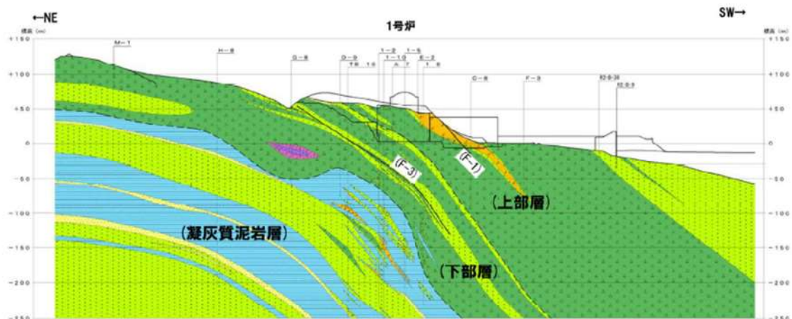
Y1-Y1' 断面
