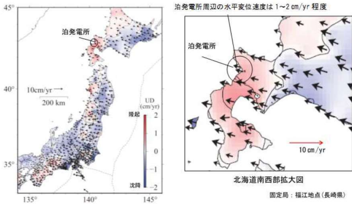
第 1.5-13 図 GEONET による 1997 年 1 月から 2000 年 1 月までの 平均変位速度 (Suito, 2018 に加筆)
