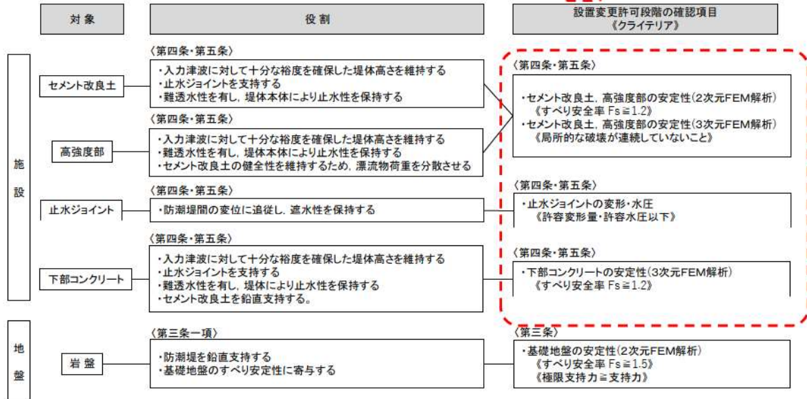
第 9-2 図 設置変更許可段階における防潮堤（標準部）の確認項目
