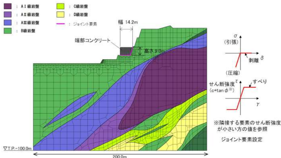
第 9-53 図 解析モデル及びジョイント要素の設定
