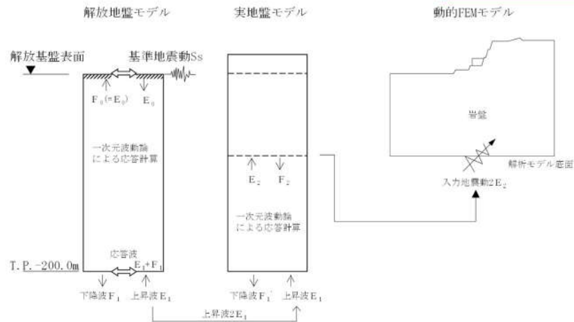
第 9-54 図 解析モデル及びジョイント要素の設定
