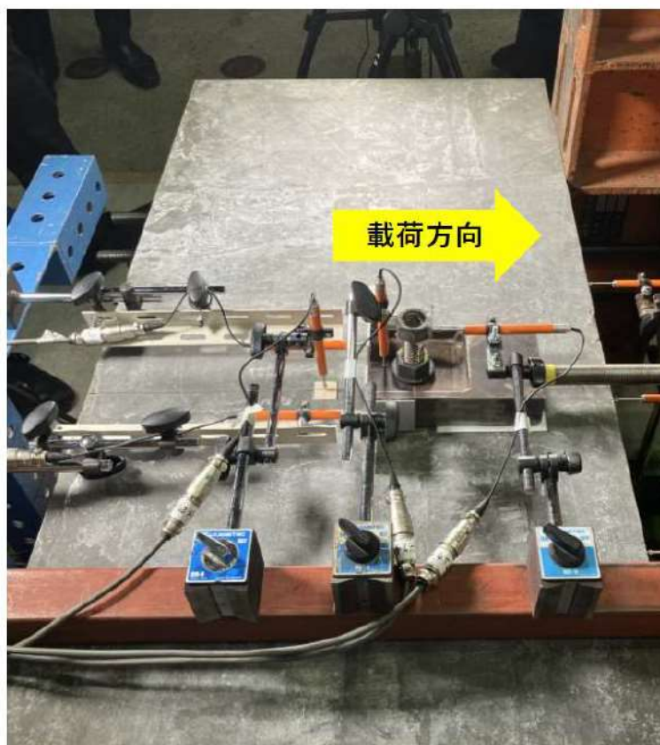
第 7-76 図 せん断試験最大荷重载荷後の状況写真（破壊形式確認ケース）
