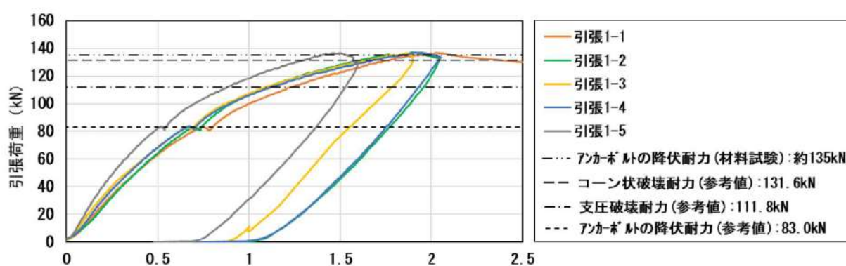
第 7-66 図 アンカーボルトの鉛直変位 (mm)
