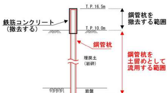
鉄筋コンクリート壁の断面図 (撤去前)
