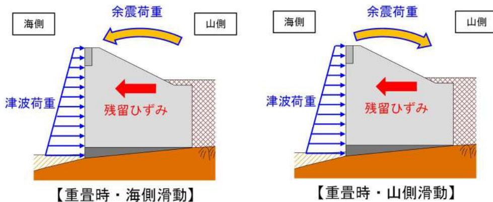
第 9-46 図 地震時の残留ひずみに対する津波荷重，漂流物荷重及び余震荷重の関係
