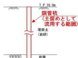
鉄筋コンクリート壁の断面図 (撤去後)
