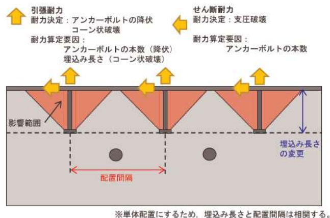
第 7-85 図 アンカーボルトの埋込み長さと配置間隔の考え方
