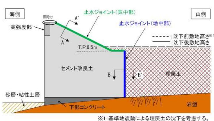
防潮堤（標準部）断面図
