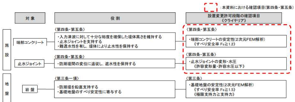
第 9-3 図 設置変更許可段階における防潮堤（端部）の確認項目
