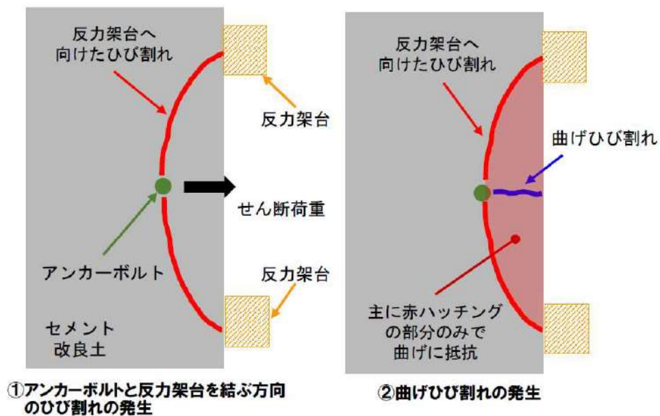
第 7-79 図 セン断供試体の破壊メカニズム
