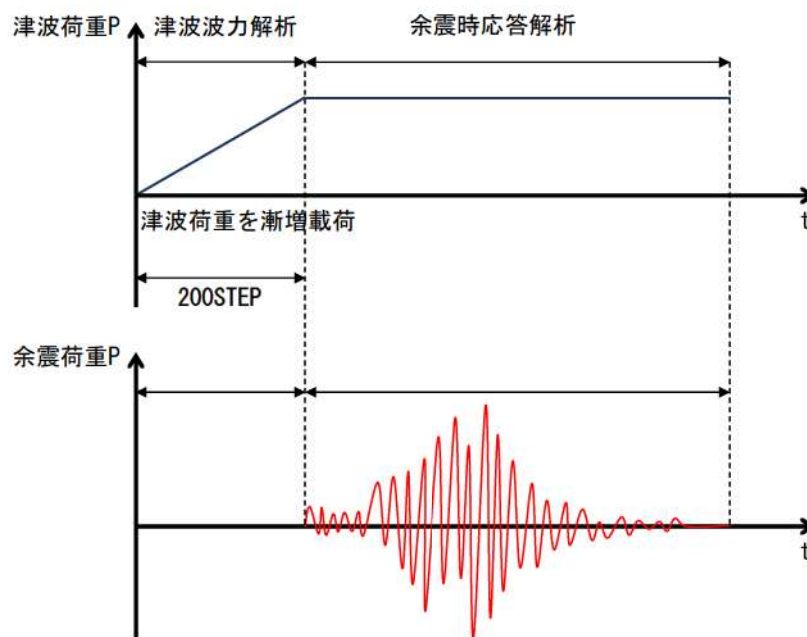
第 9-22 図 余震荷重の载荷イメージ
