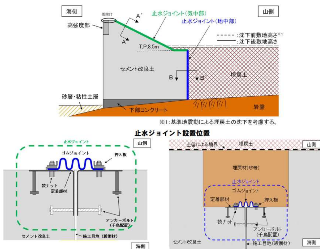
止水ジョイント（気中部）設置概要（A-A' 断面） 止水ジョイント（地中部）設置概要（B-B' 断面）
