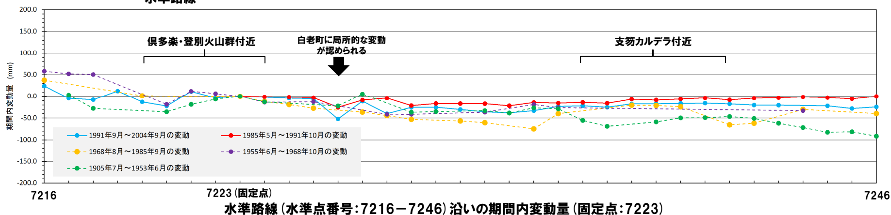
水準路線
