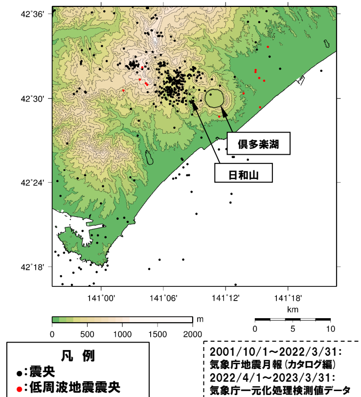
倶多楽・登別火山群周辺の震央分布図 (2001年10月1日～2023年3月31日の記録(深さ40km以浅))
