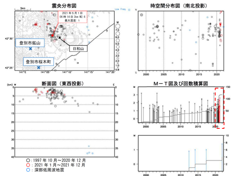
図9 倶多楽 一元化震源による周辺の地震及び深部低周波地震活動 (1997年10月～2021年12月、 M \geq 0.8 、深さ40km以浅) ・5月1日に日和山の西側で地震が一時的に増加し、そのうち日和山の西約2km、深さ3kmで発生した地震(マグニチュード2.6)により、図中に×で示した登別市鉾山及び登別市桜木町で震度1を観測しました。 ・6月以降、山体及び周辺で発生する地震は少ない状態で経過しました。
