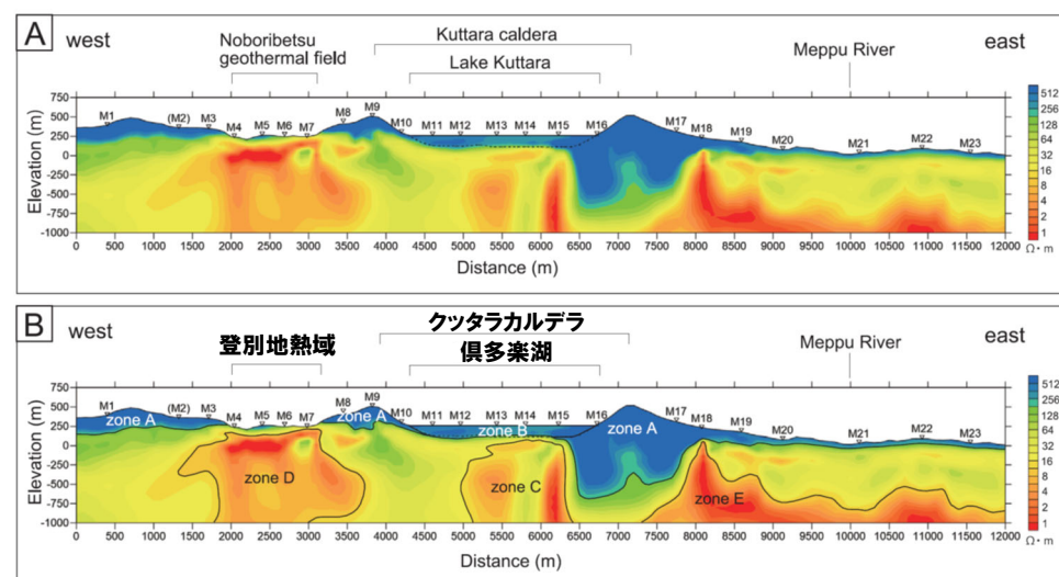
クッタラ火山直下の比抵抗構造(図A:注釈なし, 図B:注釈あり) (Goto and Johmori (2015) に加筆)
