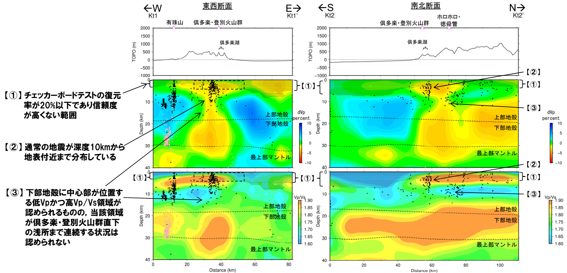
地震波速度構造 (鉛直断面, 断面位置図はP409参照)
