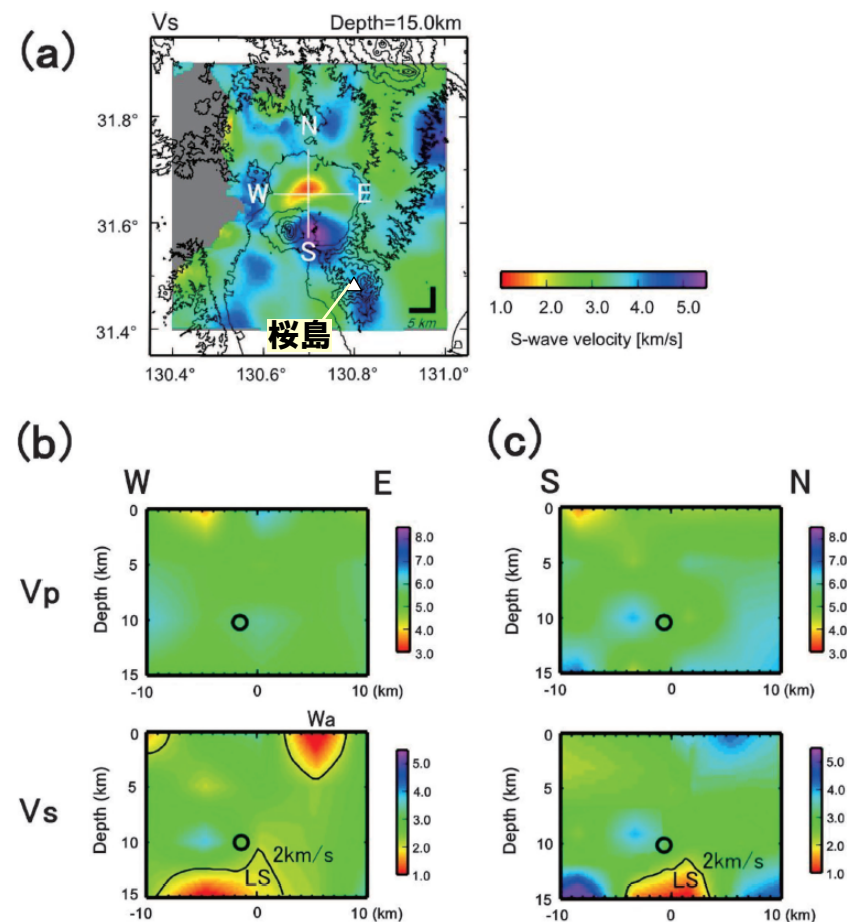
(a) 震度15kmにおけるVs断面 (b) (c) Vp及びVsの東西及び南北方向の鉛直断面 (為栗ほか (2022) に加筆)
