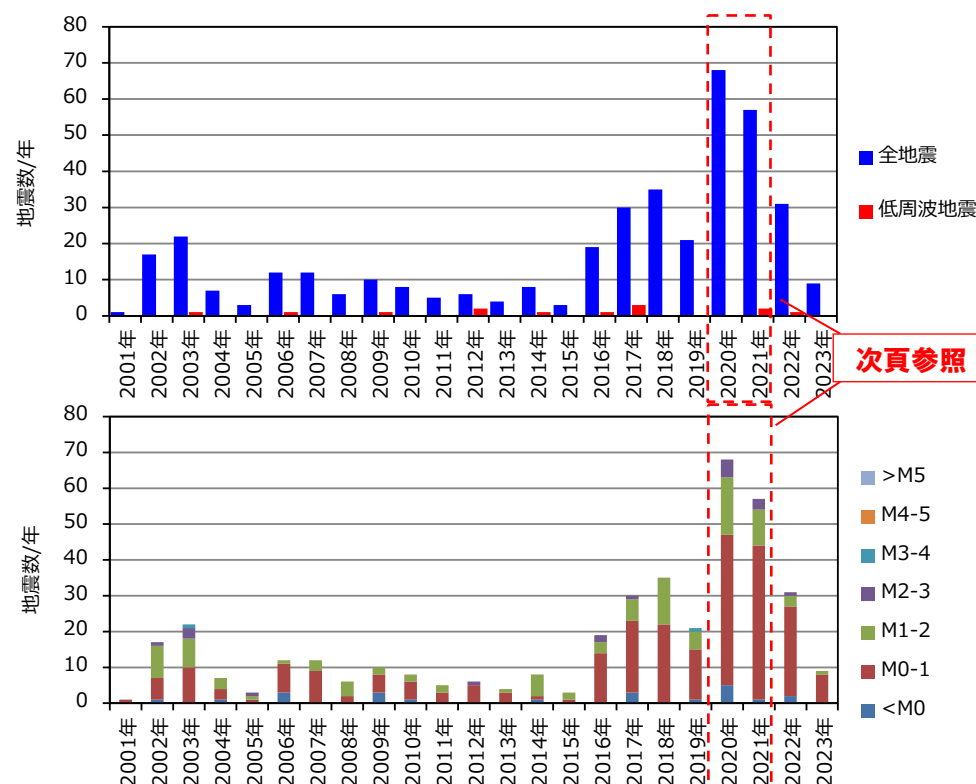
地震発生回数の年別時間変化(2001年～2023年※, 深さ40km以浅)
