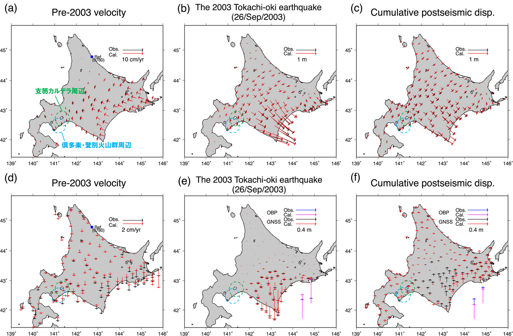
GNSS及びOBPによる2003年十勝沖地震前、地震時及び地震後の地殻変動 (a~c: 水平変位, d~f: 鉛直変位, 黒矢印が観測値, 赤矢印が計算値) (Itoh et al. (2019) に加筆)
