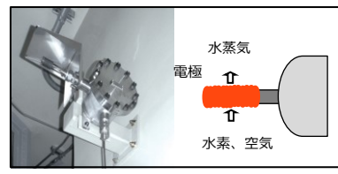
格納容器水素イグナイタ
