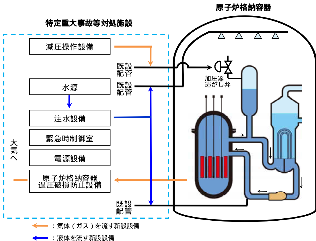
特定重大事故等対処施設概念図
