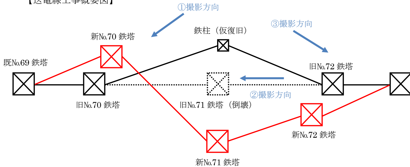
【送電線工事概要図】
