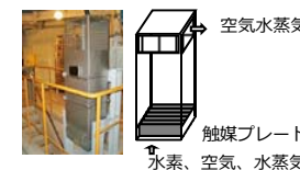
格納容器内水素処理装置(PAR)
