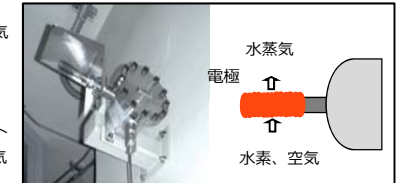
格納容器水素イグナイタ
